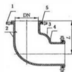
e) 弯头突面法兰密封 XT WRF 1 *
