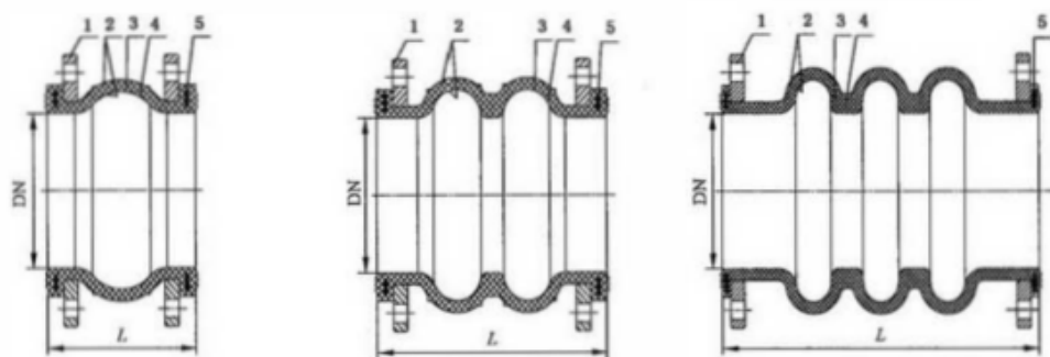
a) 单球体突面法兰密封 XT Q 2 RF 2 * b) 双球体突面法兰密封 XT Q 2 RF 2 * c) 三球体突面法兰密封 XT Q 2 RF 2 *
