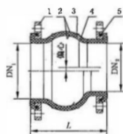
g) 单球体突面法兰密封偏心异径 XT Q 1 Y 2 RF 1 *
