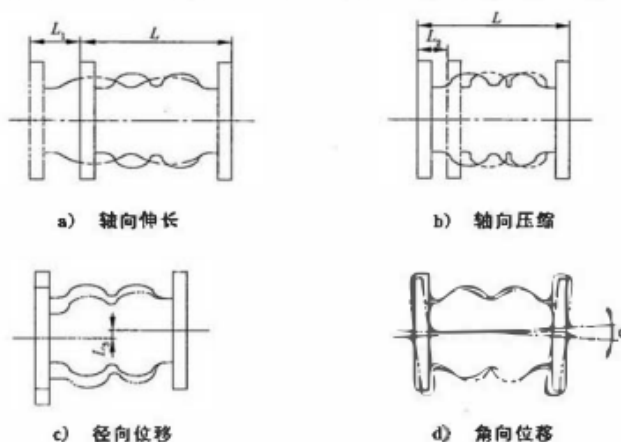
图 1 可曲挠橡胶接头的位移
